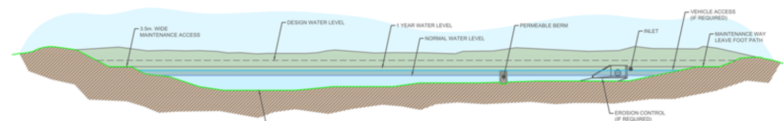
LONGITUDINAL SECTION A-A SCALE 1:200
